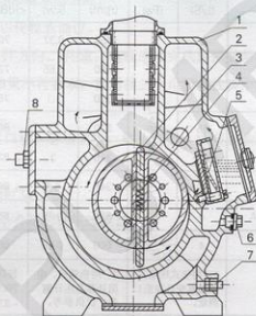
2X-30A 2X-70A结构原理图
