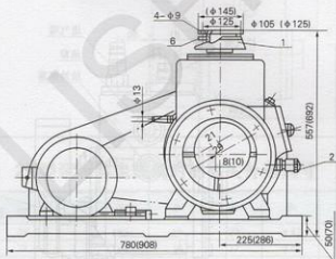
2X-30A, 2X-70A型
