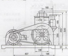
2X-8, 2X-15型
