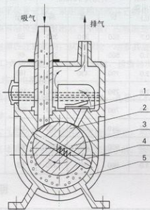
2X-2A 2X-4A 2X-8 2X-15结构原理图
